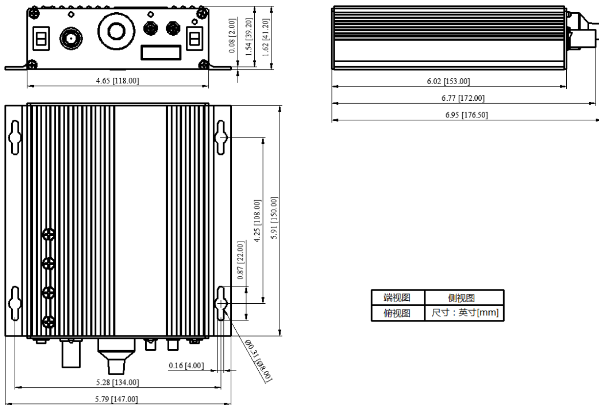
图5、AHVA100V2X5MA的尺寸图
