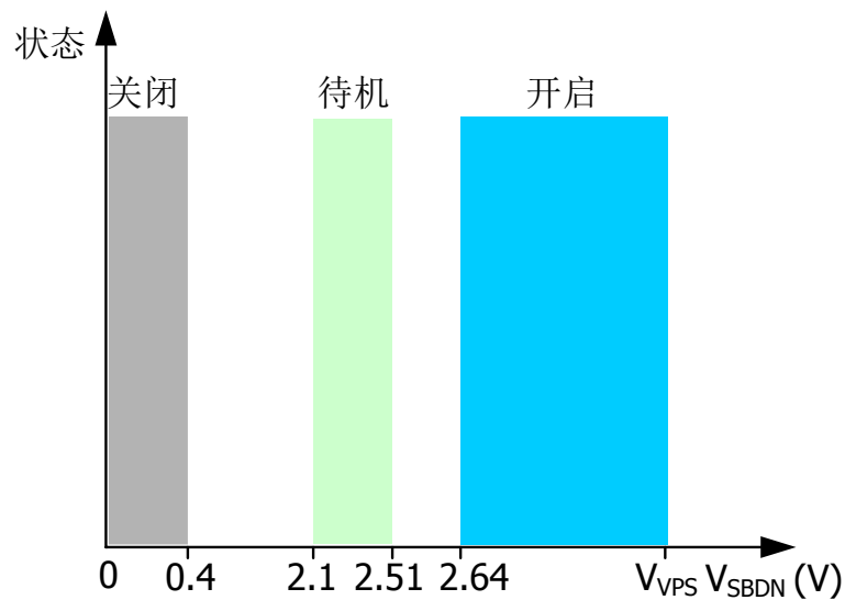
图 3、 V_{SDN} vs. 放大器状态
