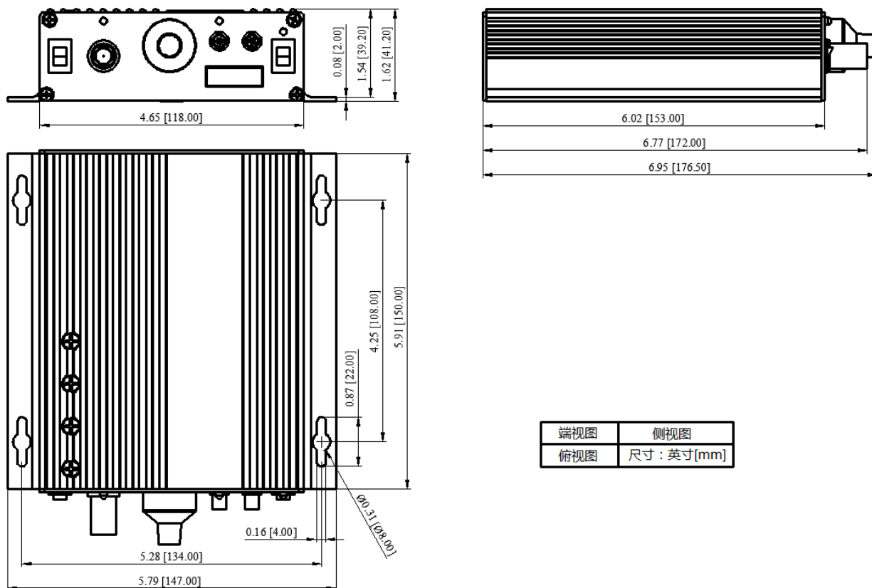
图11、AHVA250V2X100MA的尺寸图
