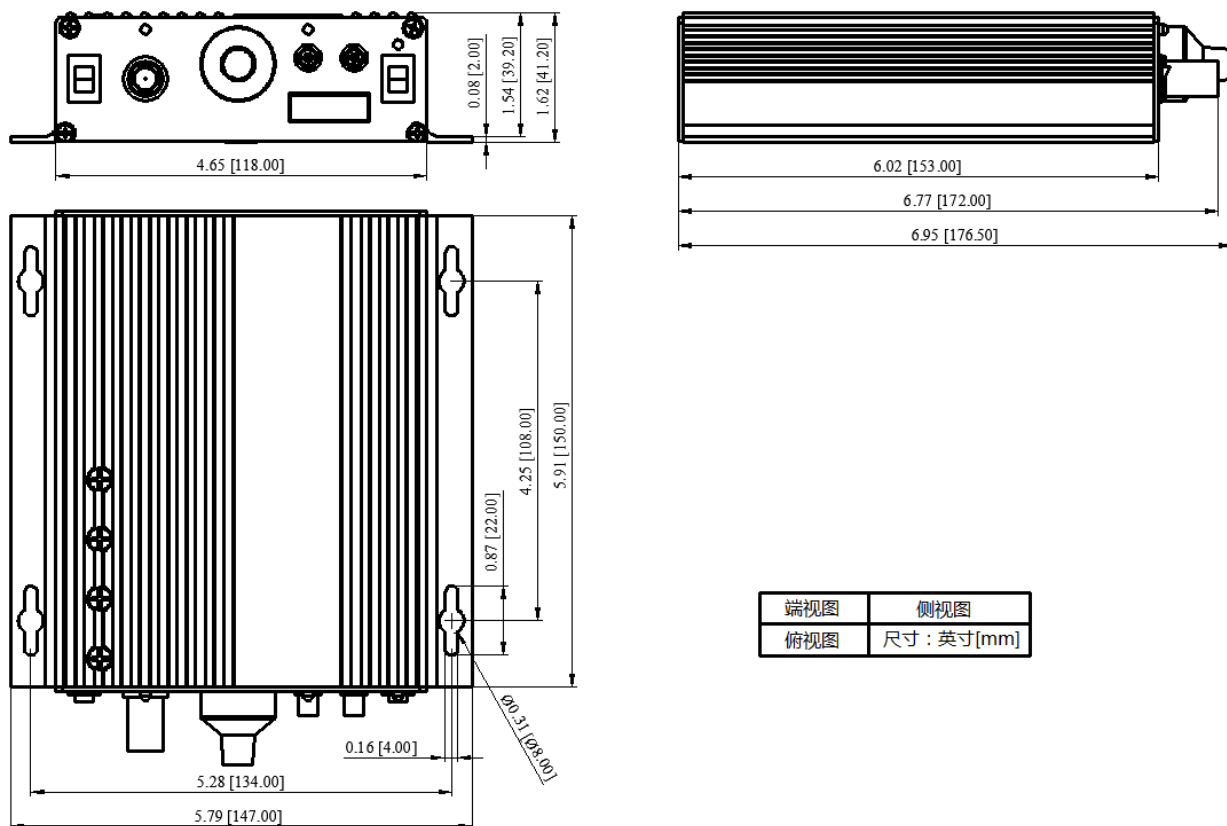
图11、AHVA250V2X5MA的尺寸图
